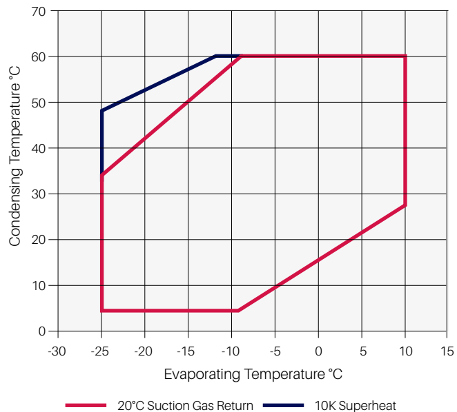
ZB - R448A/R449A
