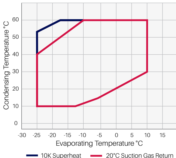
YBD*1E - R454A
