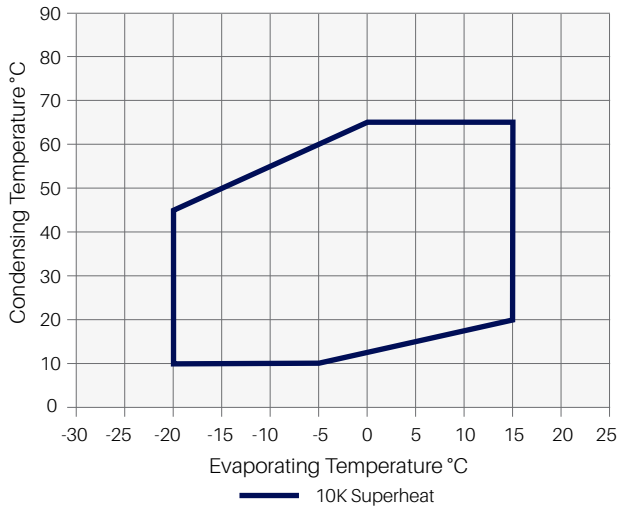
ZRD - R513A
