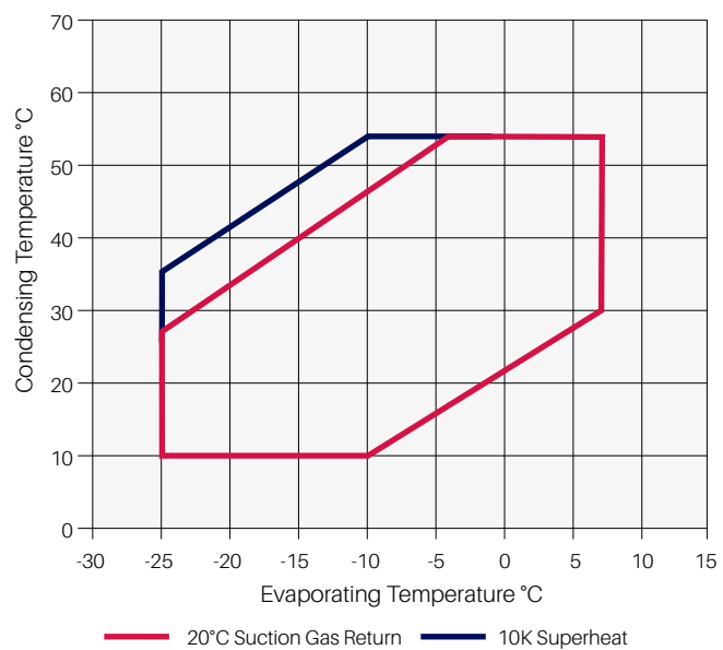
ZB - R407A
