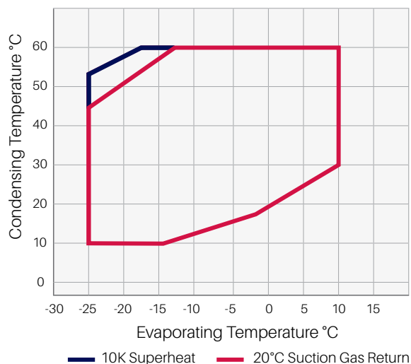
YBD*1E - R455A
