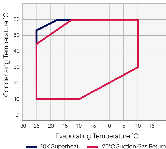
YB*1E - R455A
