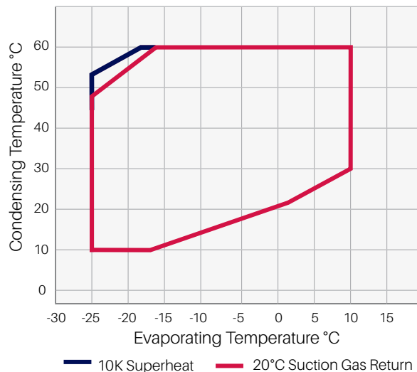
YBD*1E - R454C
